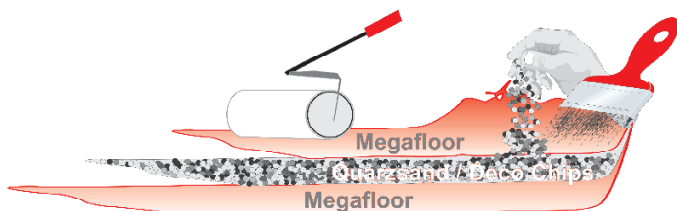
Schichtaufbau Megafloor System
