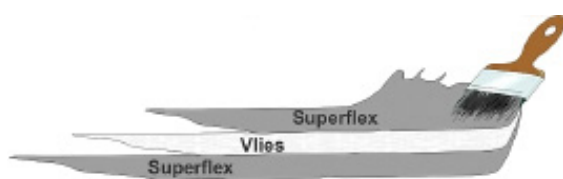
Schichtaufbau Superflex System
